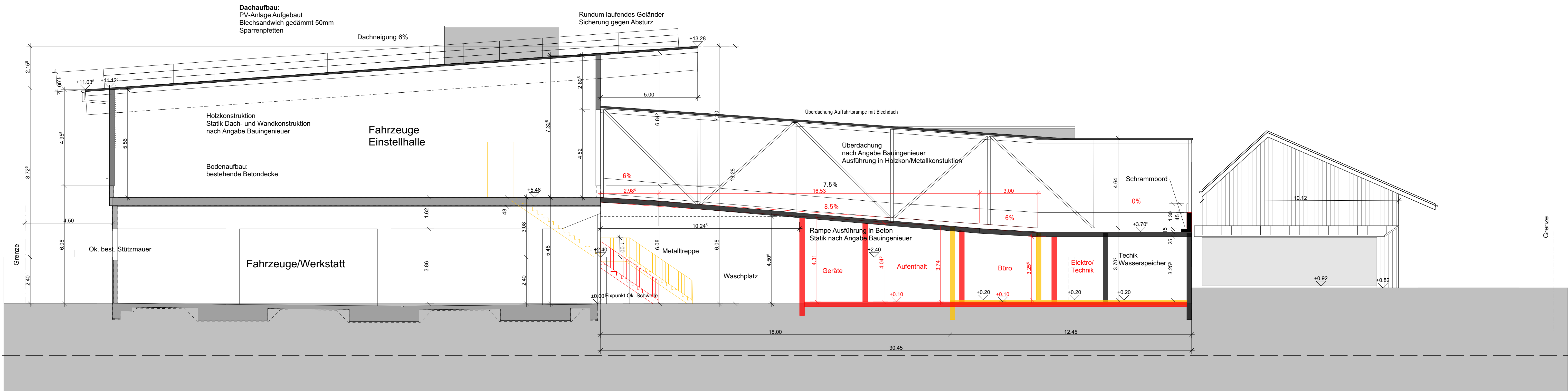
Schnitt 4
