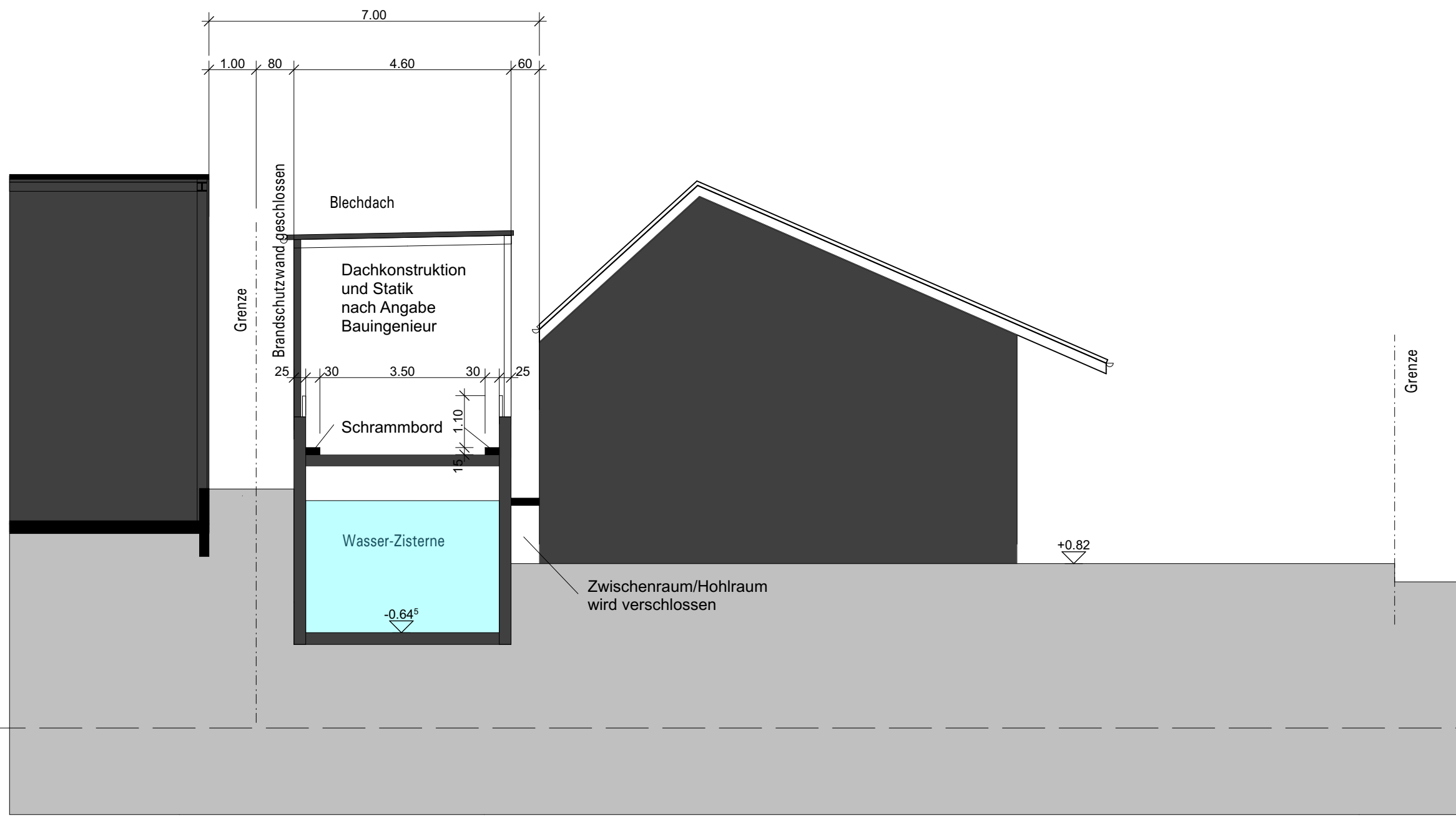
Schnitt 5
