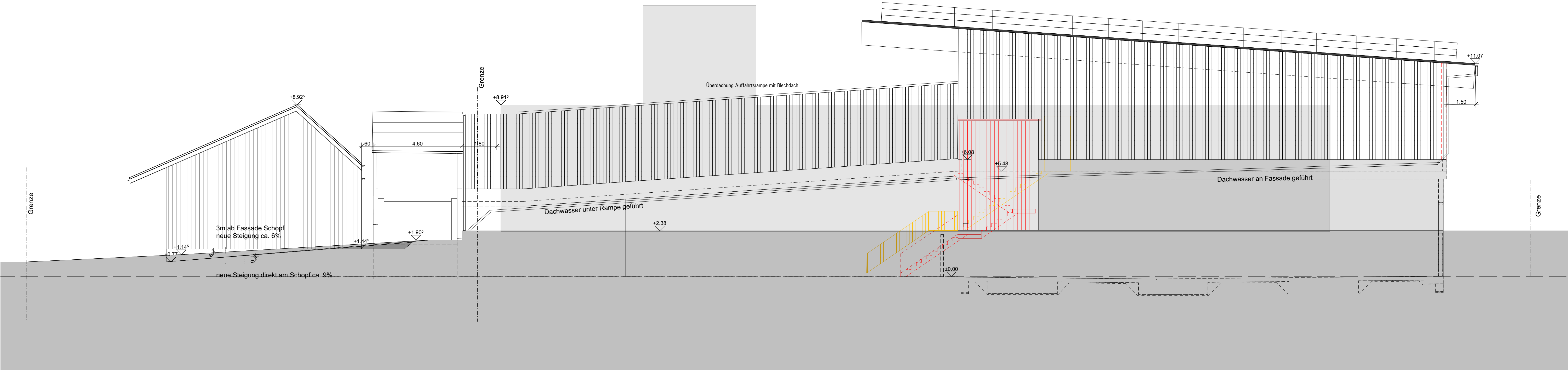
Ansicht West (Schnitt an Fassade Schopf)
