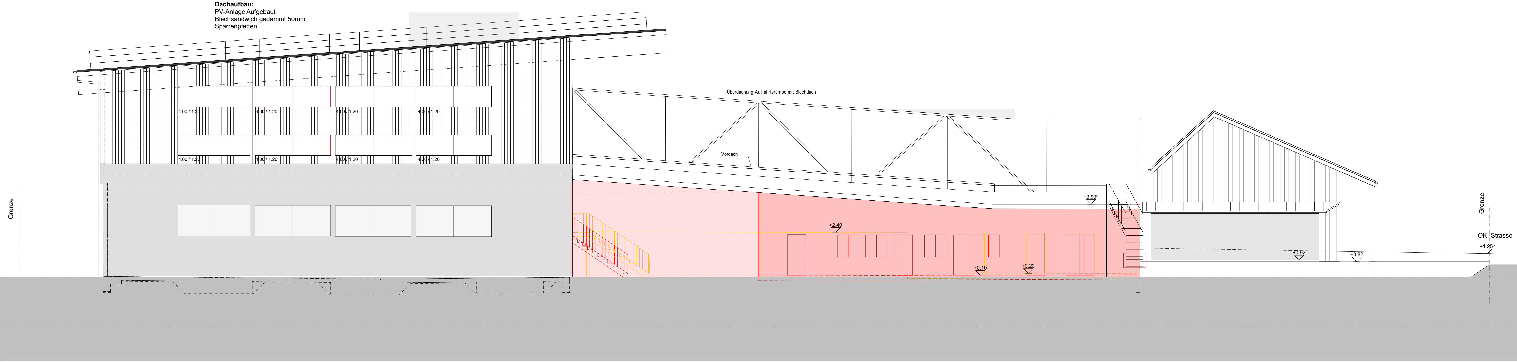
Ansicht Ost
