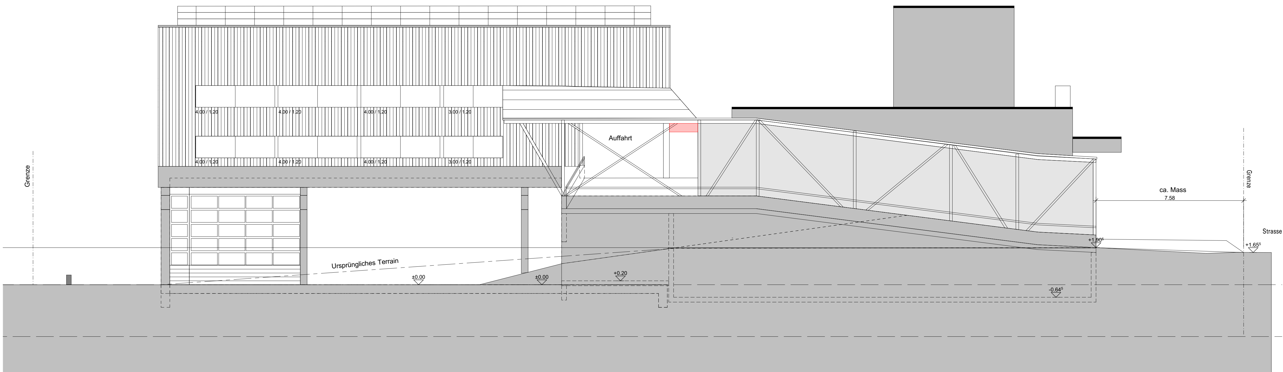
Ansicht Nord
