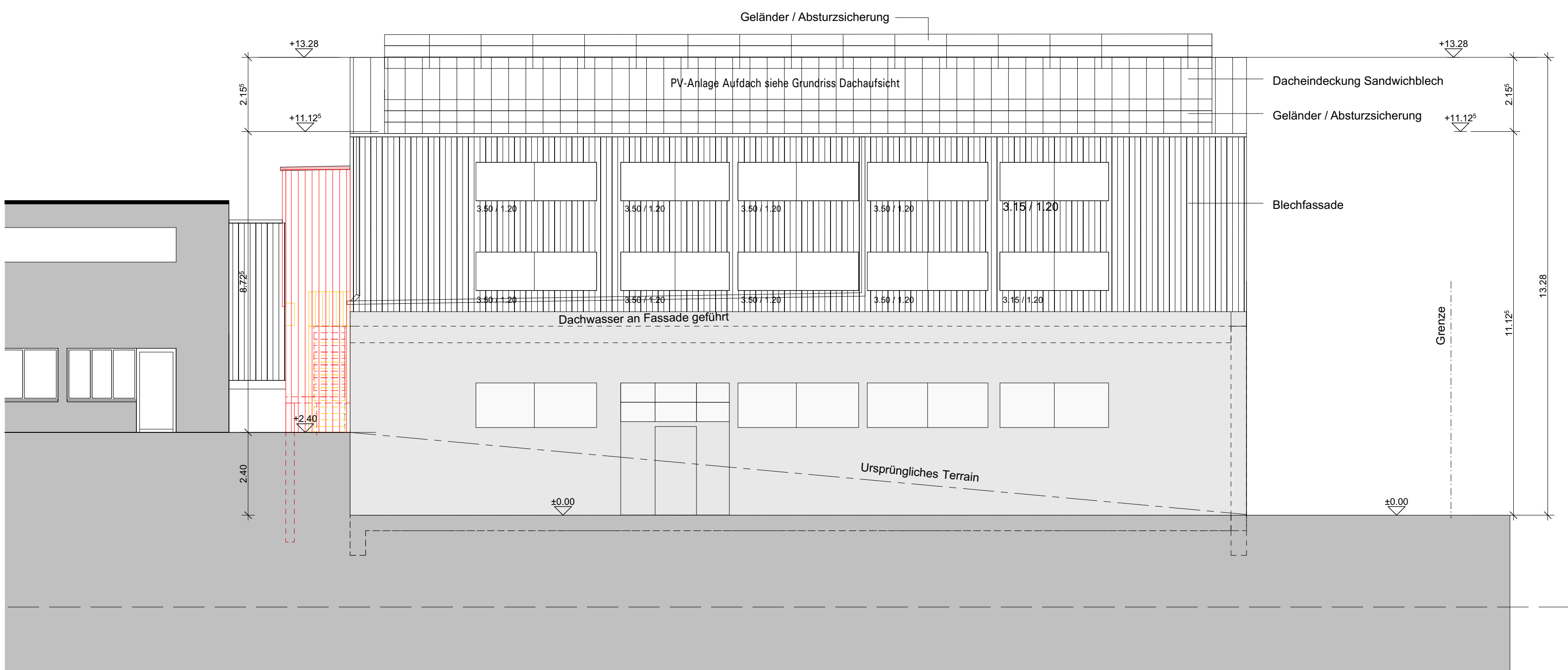
Ansicht Süd
