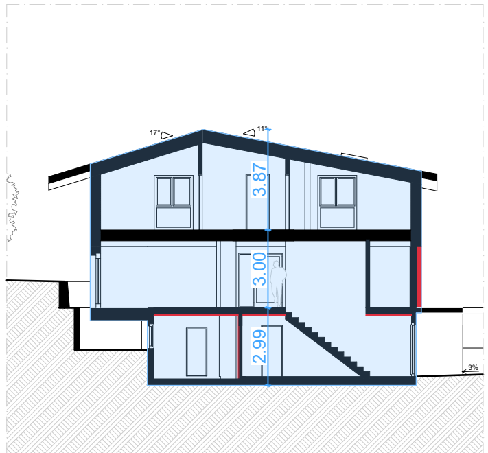
Schnitte AA
