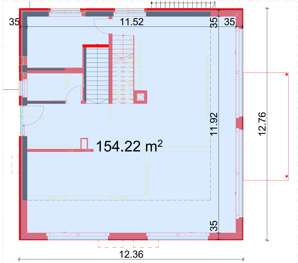
Erdgeschoss
