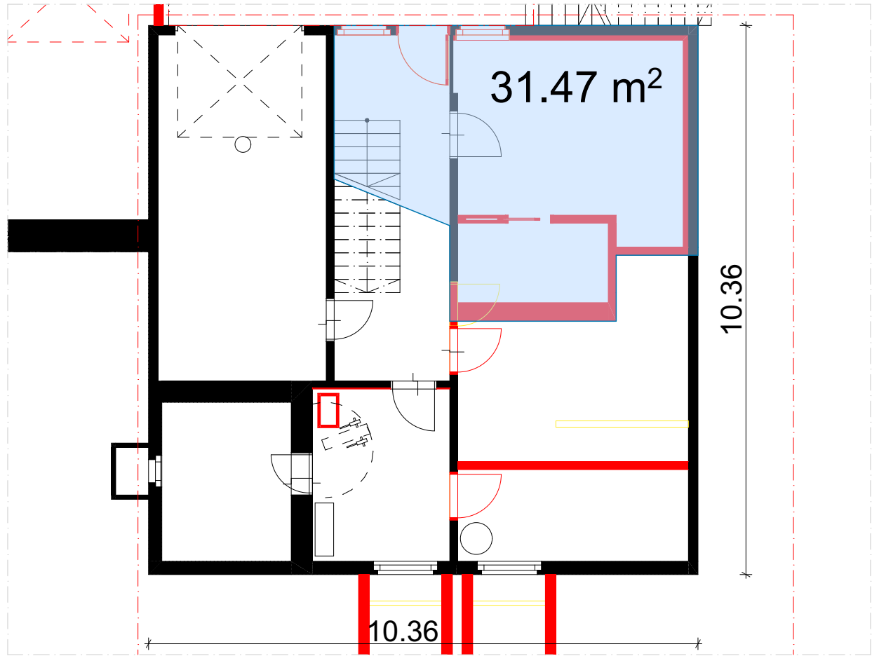
Untergeschoss
