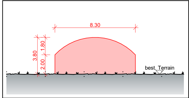
Schemaschnitt Folientunnel, 1:200
