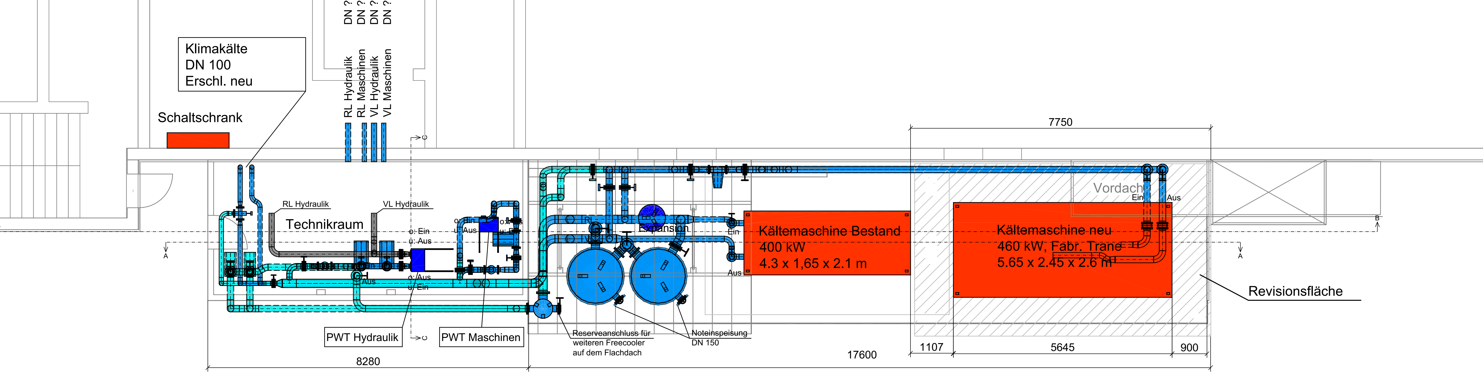
Grundriss
