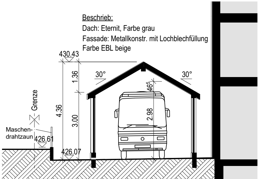
Schnitt Carport
