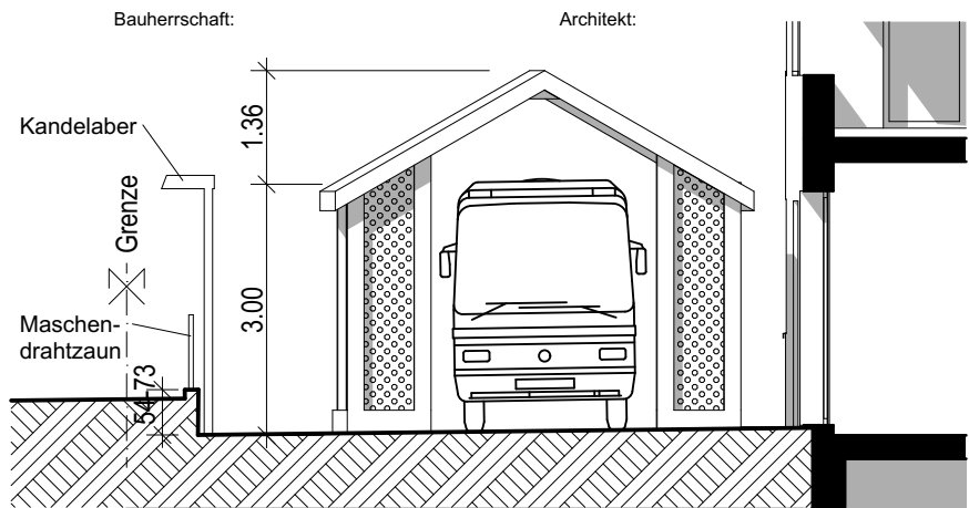
Ansicht Ost
