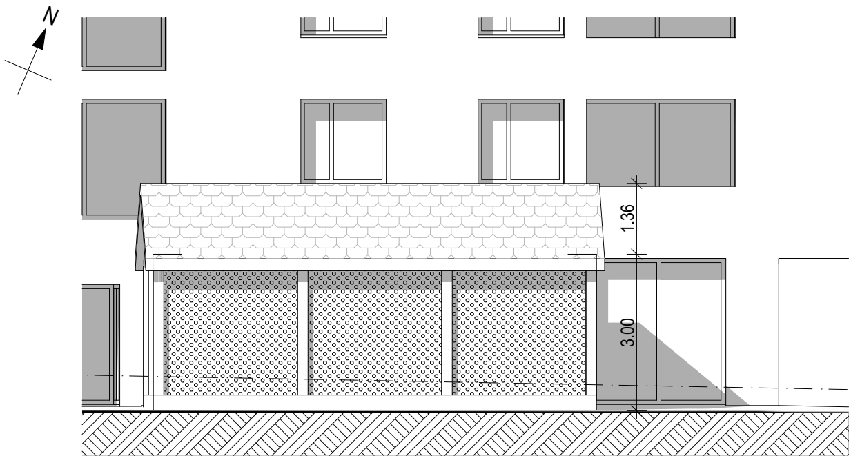
Ansicht Süd
